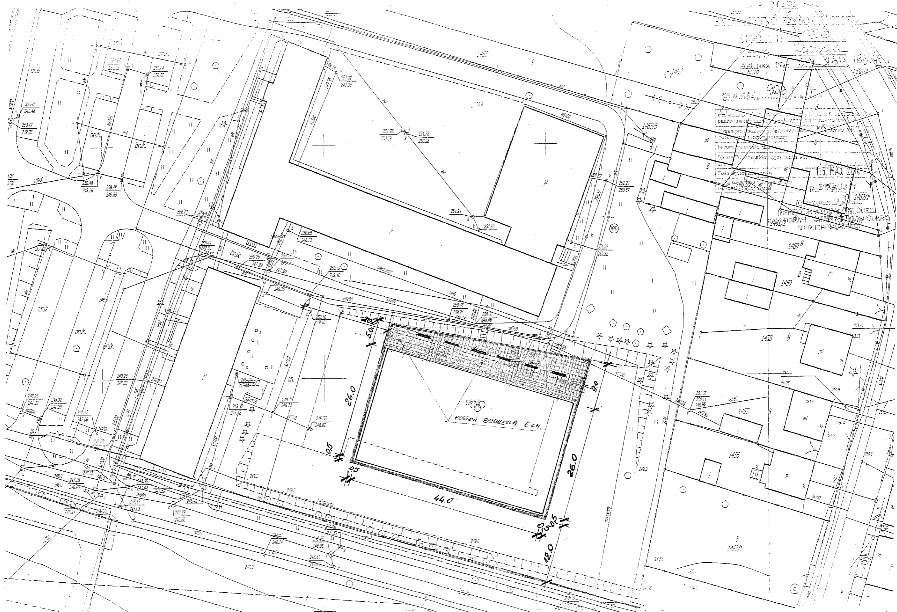
REMONT BOISKA SPORTOWEGO WIELOFUNKCYJNEGO PRZY ZG NR 3 W KŁOBUCKU UL. SKORUPKI 48 SZKIC SYTUACYJNY Kwiecień 2014 Rys. nr 1
