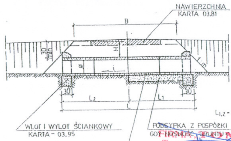
PRZEKRÓJ PODŁUŻNY
