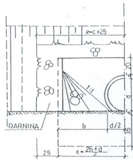
PRZEKRÓJ PODŁUŻNY
