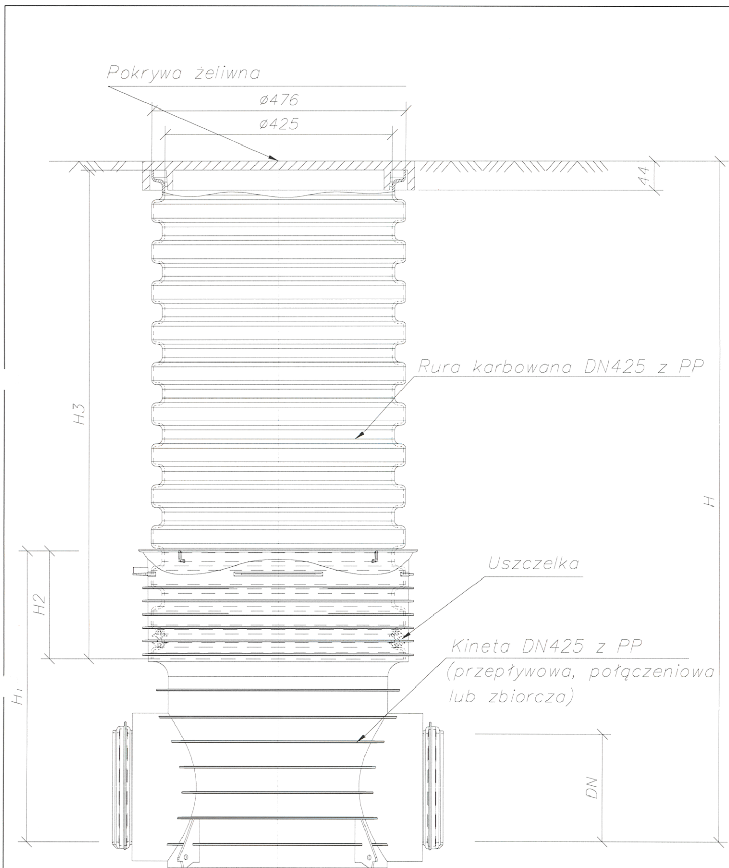
Studzienka inspekcyjna DN425 z rur PP karbowanych z pokrywą żeliwną
